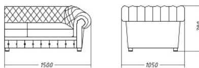
модуль диван двухместный с 1 подлокотником
