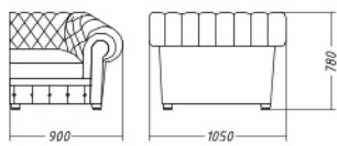
модуль кресло с одним подлокотником
